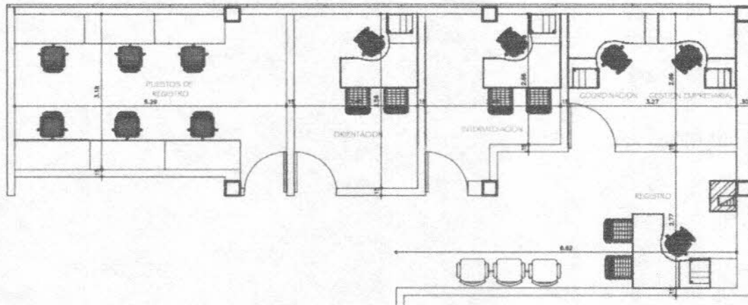
Figura 3. Planos Piso 2
